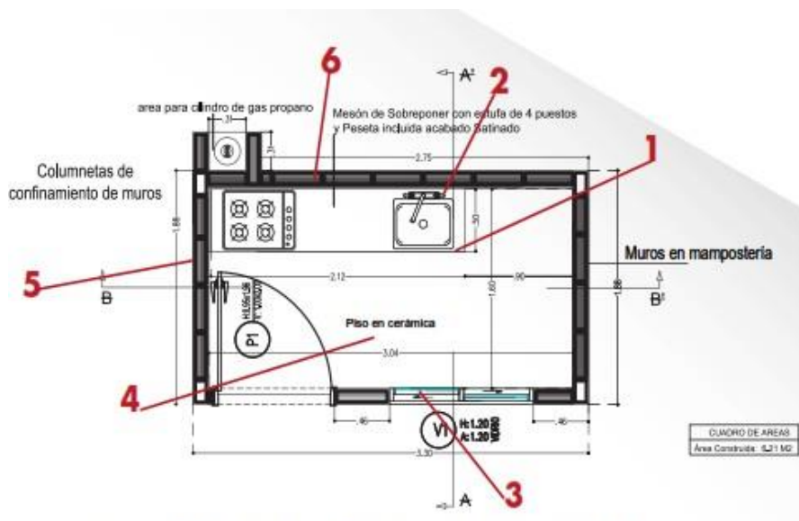
PLANTA ARQUITECTONICA TIPO C - 1.1
