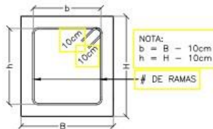
DET. ESTRIBOS CIMENTACION Esc.: 1:75
