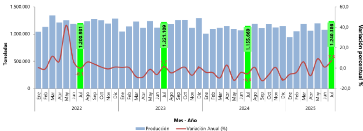
Gráfico 5. Producción de cemento gris (toneladas y variación anual de la producción) Enero 2022 – julio 2025 p
