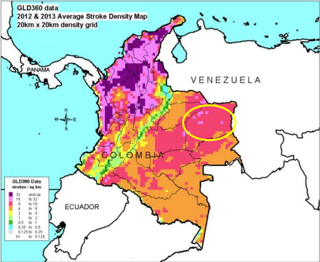
Densidad Promedio de Descargas Eléctricas por Km2.
