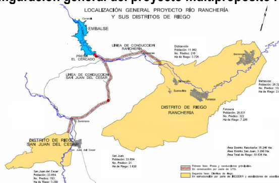
Figura. Configuración general del proyecto multipropósito río Ranchería
