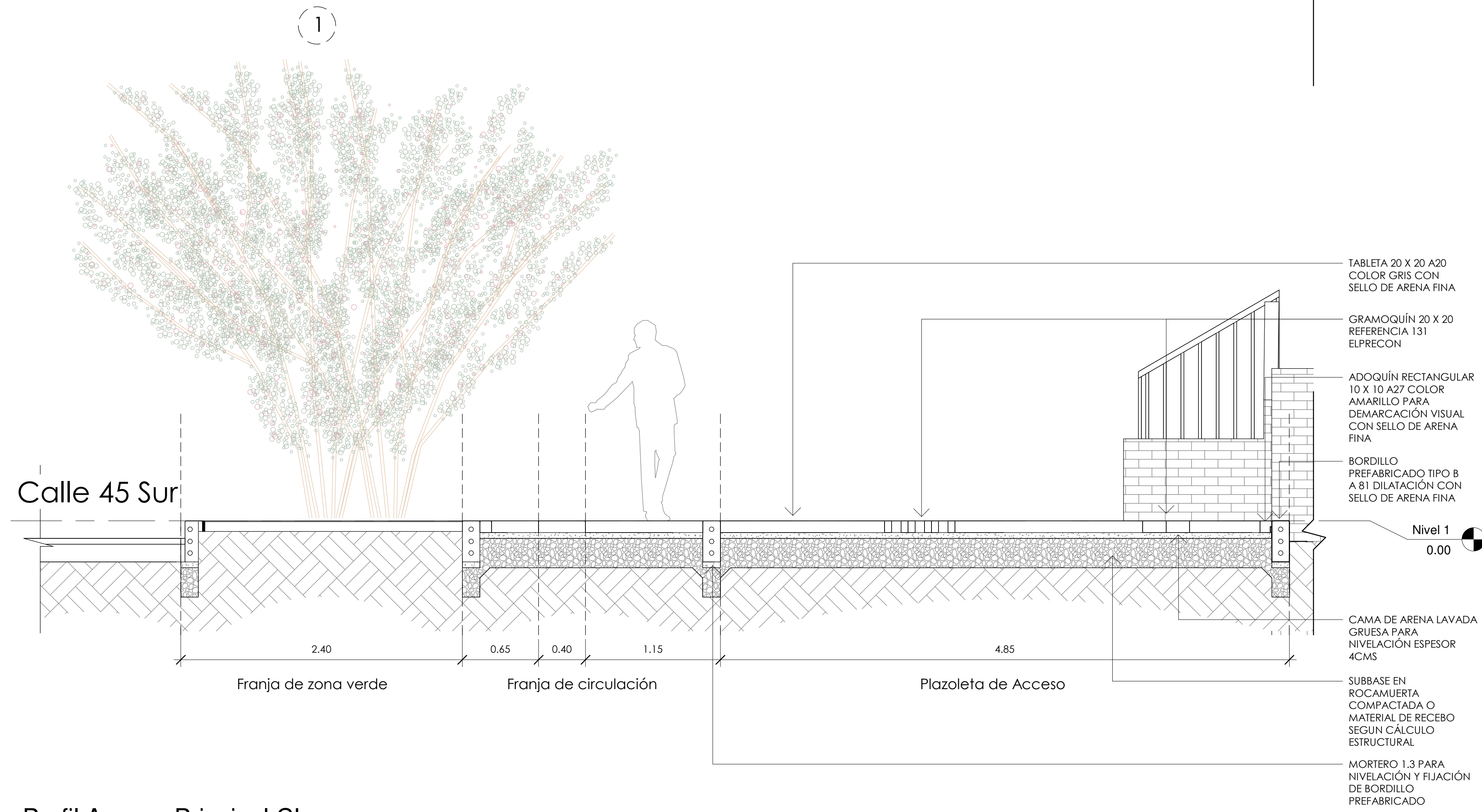
2 Perfil Acceso Principal CL 45SUR 1 : 25
