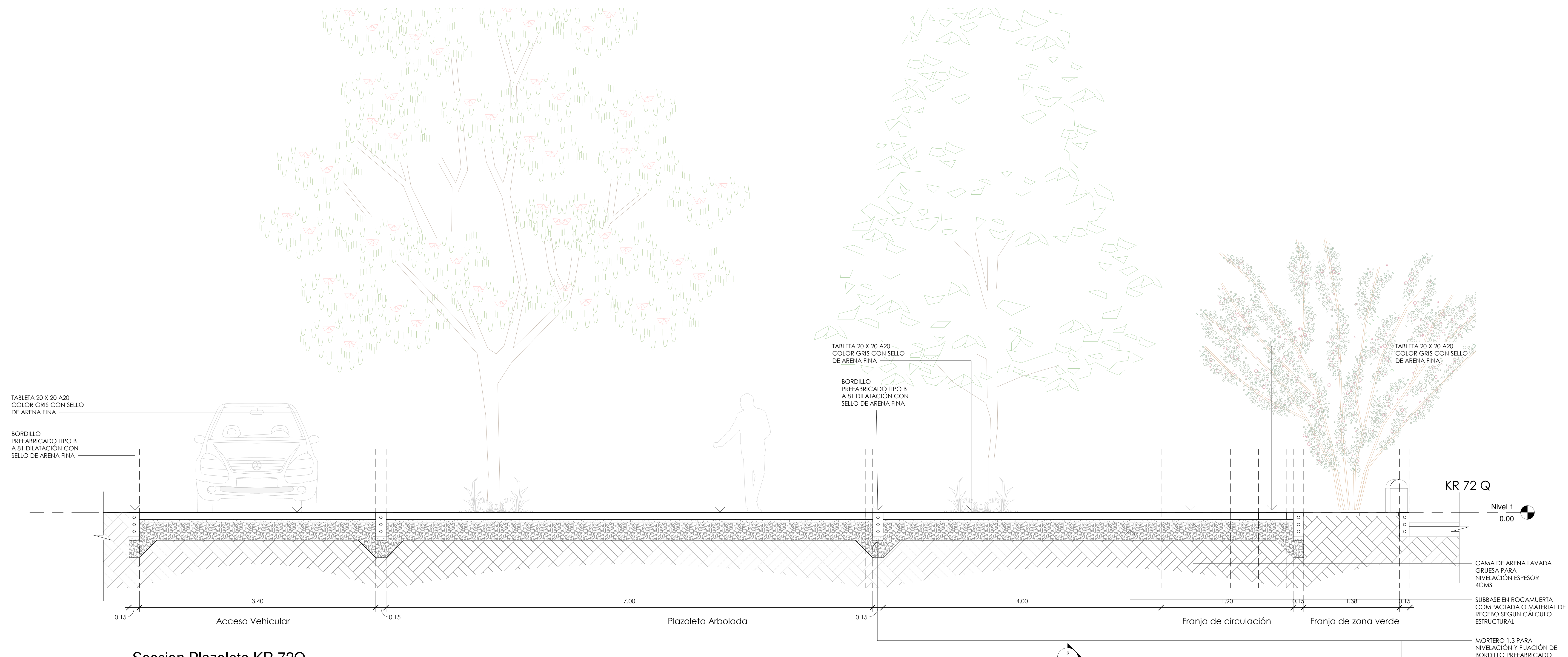
2 Seccion Plazoleta KR 72Q 1:25
