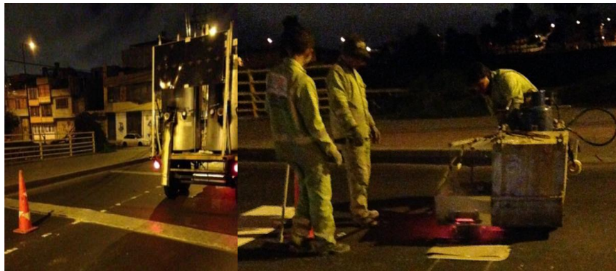
Gráfico 39. Máquinas de aplicación de resina termoplástica
