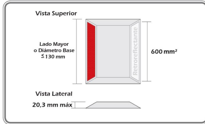
Gráfico 11. Tachas Reflectivas
