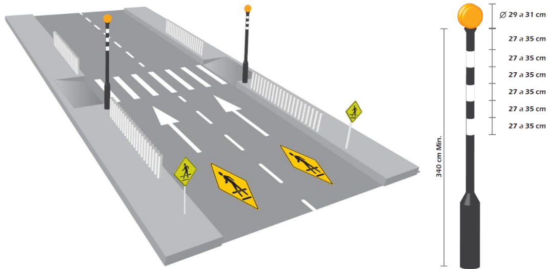
Fuente: Manual de Señalización Vial 2015 figuras 6.1-2 y 6.1-4
