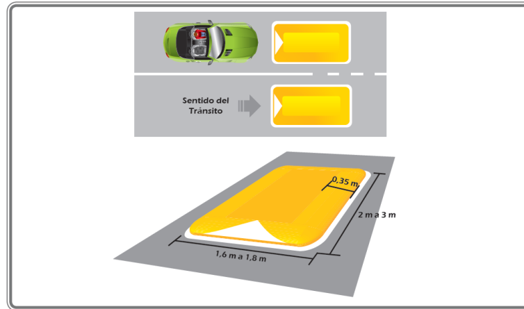
Fuente: Manual de Señalización Vial 2015 Figura 5-29
