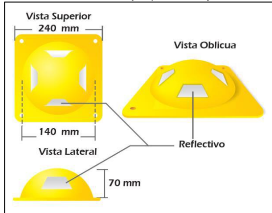
Gráfico 14. Ejemplos de Boya
