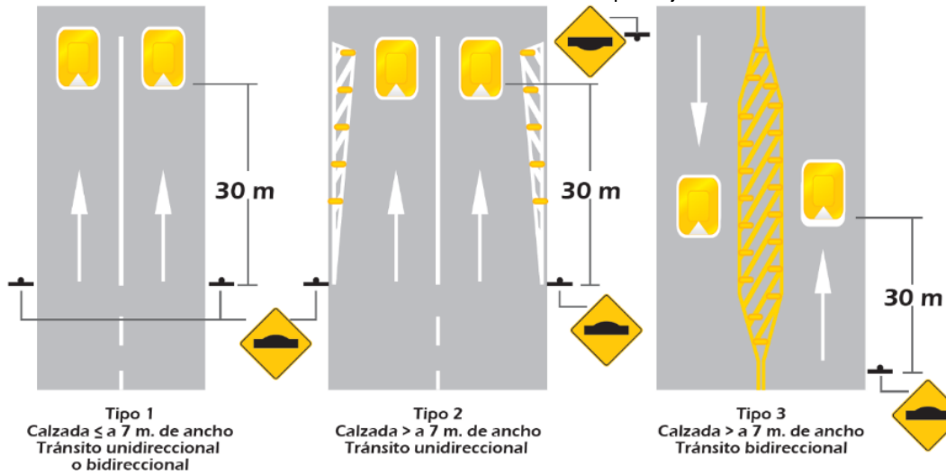
Gráfico 23. Ubicación de Resaltos Tipo Cojín
