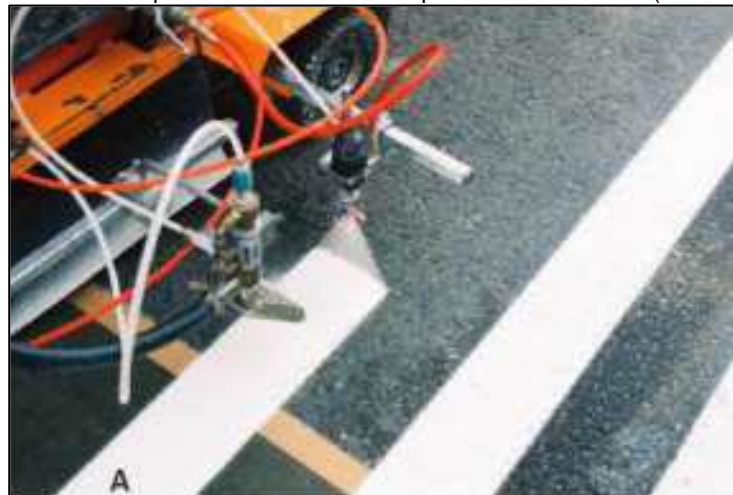
Gráfico 37. Aplicación con sistema de pulverización sin aire (Airless)
