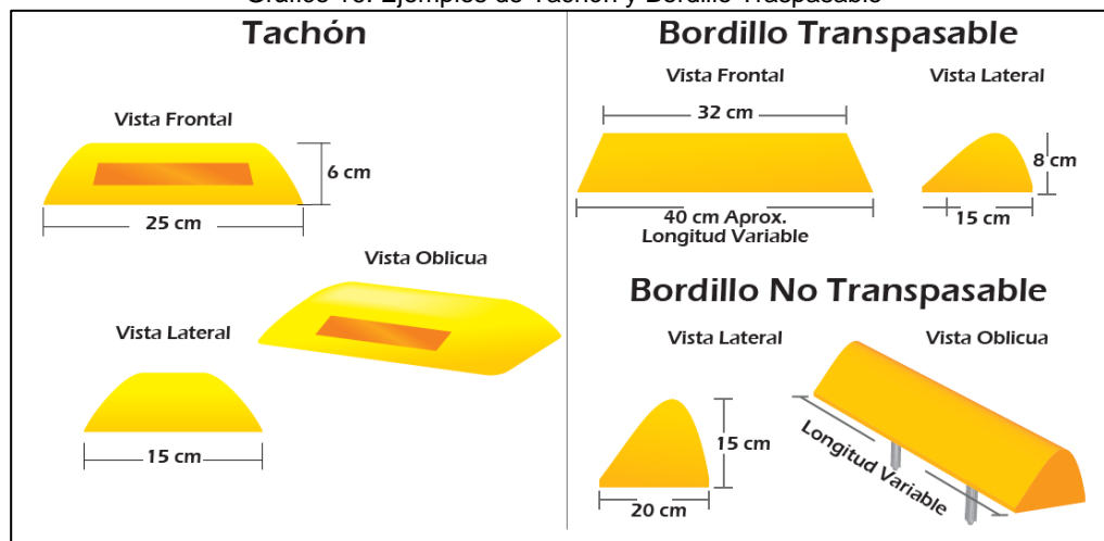
Gráfico 16. Ejemplos de Tachón y Bordillo Traspasable
